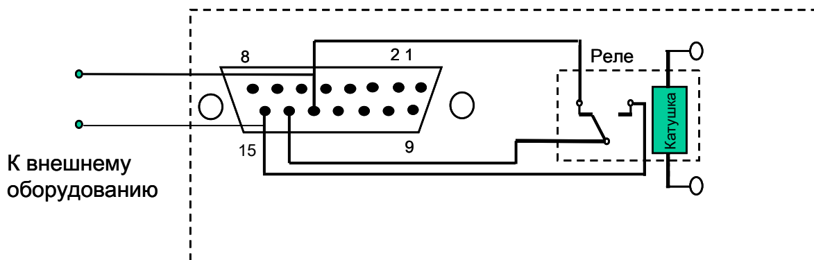
Нормально открытое подключение (выводы 13 и 14)
