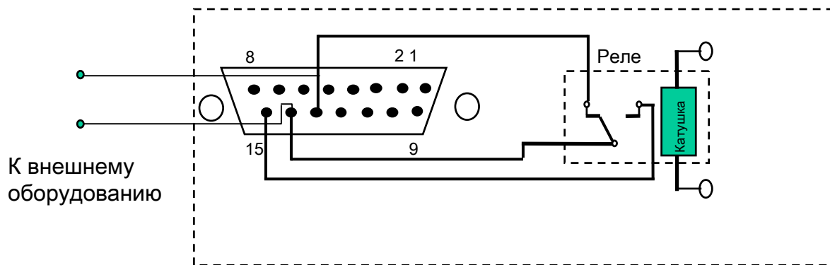
Нормально закрытое подключение (выводы 13 и 12)
